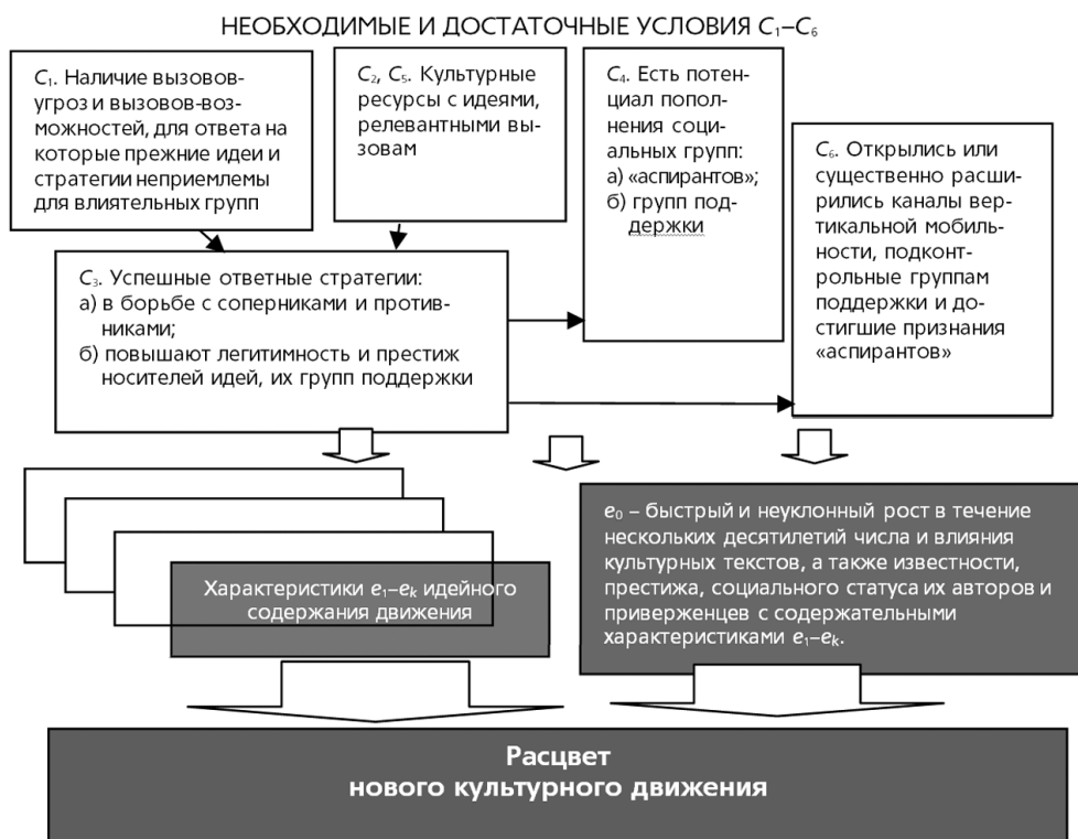
Рис. 1. Логическая схема следствия суждения о макрособытии E «расцвет культурного движения» из суждений о комплексе необходимых и достаточных обстоятельств ( C_1, \dots, C_n ).
